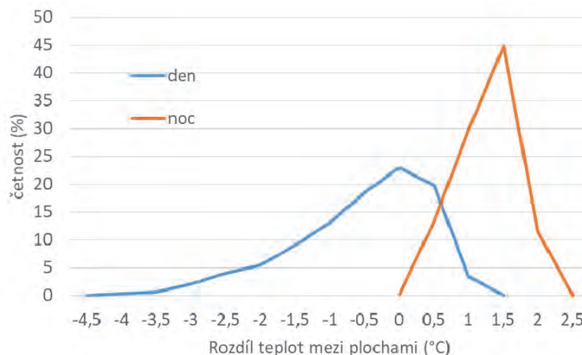
Obr. 1: Rozdělení četností rozdílů přízemních teplot vzduchu mezi variantami kontrola a C5.
